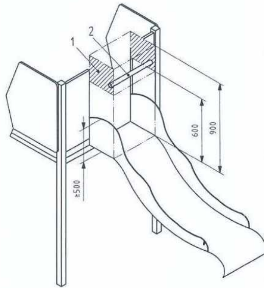
a) 1 000 mm 초과높이의 부착미끄럼틀 출발지점 측면보호대와 가로대의 적합한 위치의 보기
