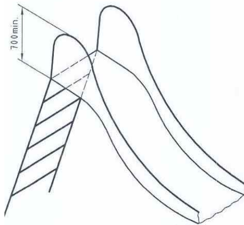
b) 독립미끄럼틀 출발지점의 측면보호대의 보기 <그림 1> 측면보호대의 보기
