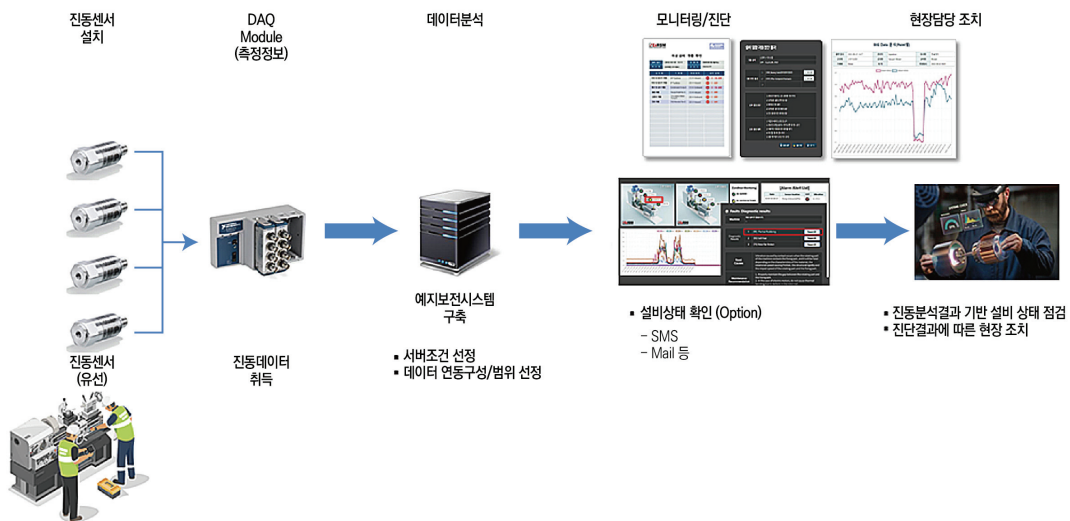
〈그림 1〉 진동센서 설치, 데이터 취득 및 사용자 조치 프로세스 구성도
