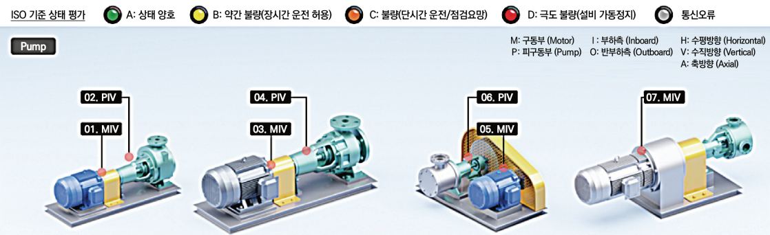
〈그림 3〉 모터+펌프적용 설비 데이터 취득 사례
