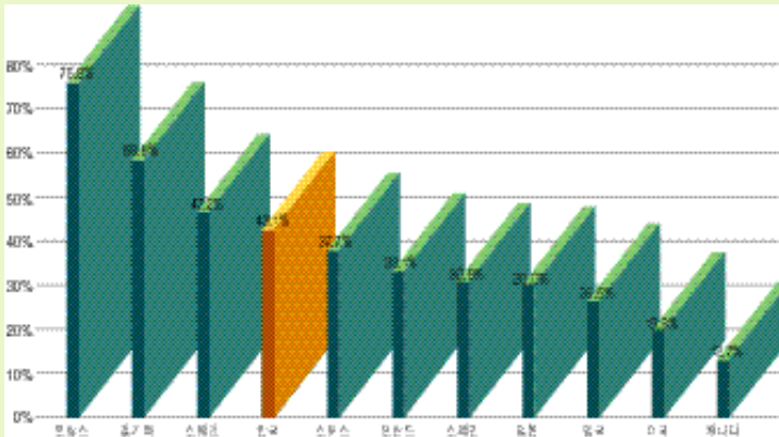
전체발전량중원자력발전비중 (1999)
