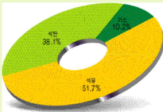
CO 2 배출량 (2000)
