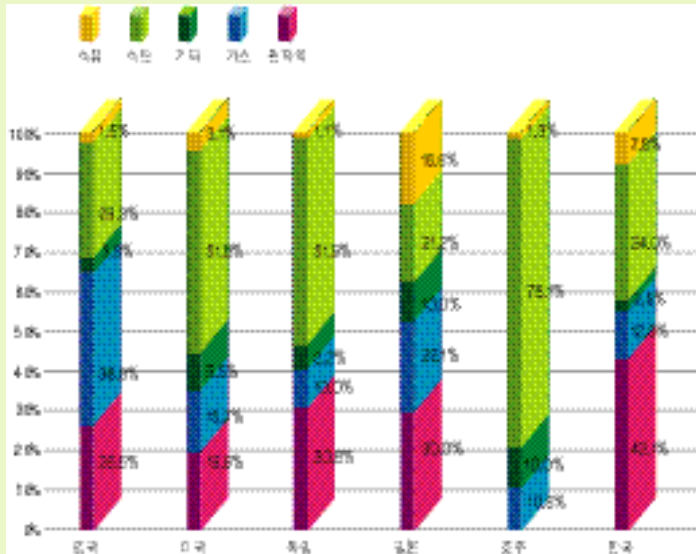
전원구성비 (1999)
