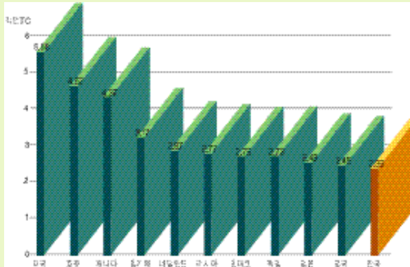
주요국의1인당CO 2 배출량 (1999)
