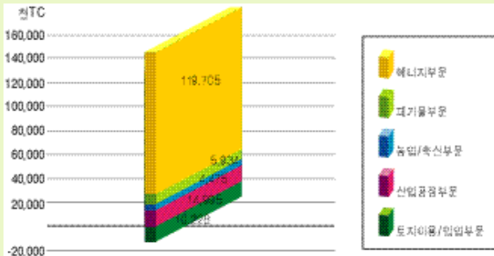
부문별 온실가스 배출량 (2000)
