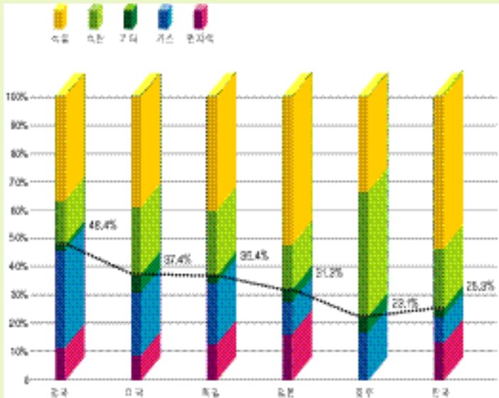
에너지원중청정에너지비중 (1999)
