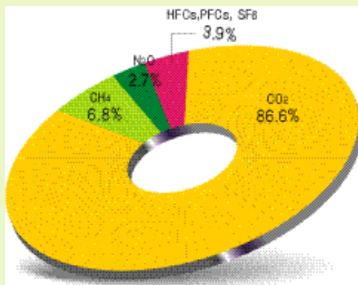
온실가스별배출구성 (2000)
