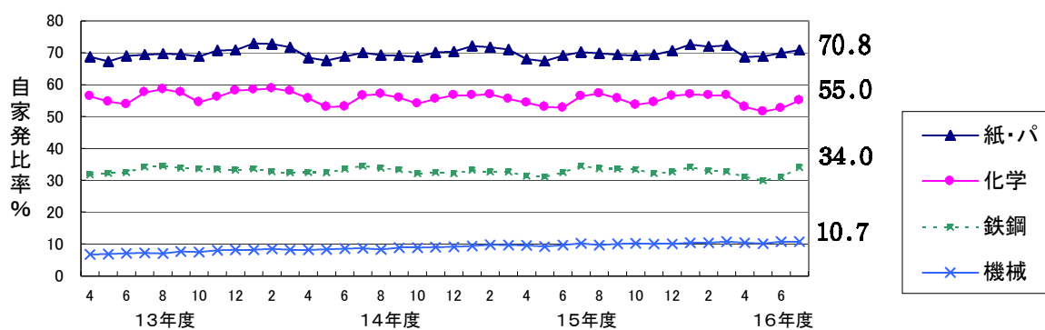
大口需要の業種別自家発比率の推移
