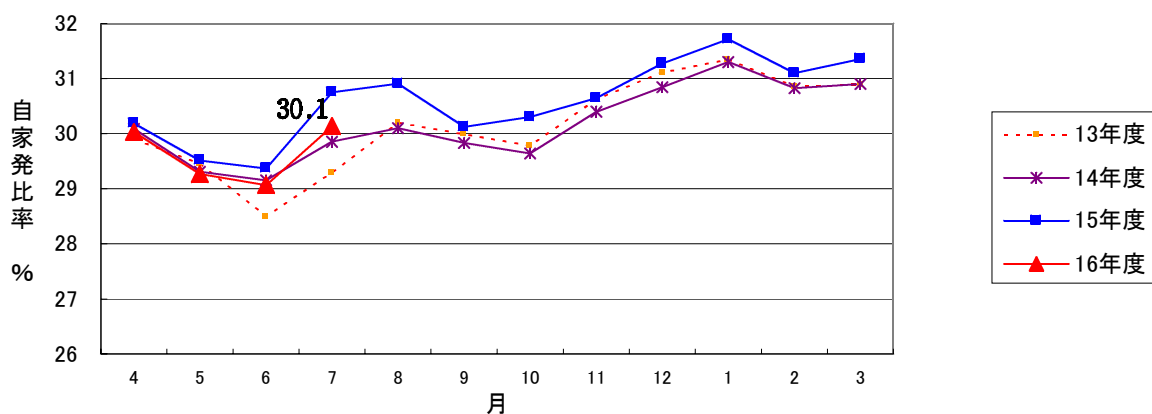
大口需要の自家発比率の推移
