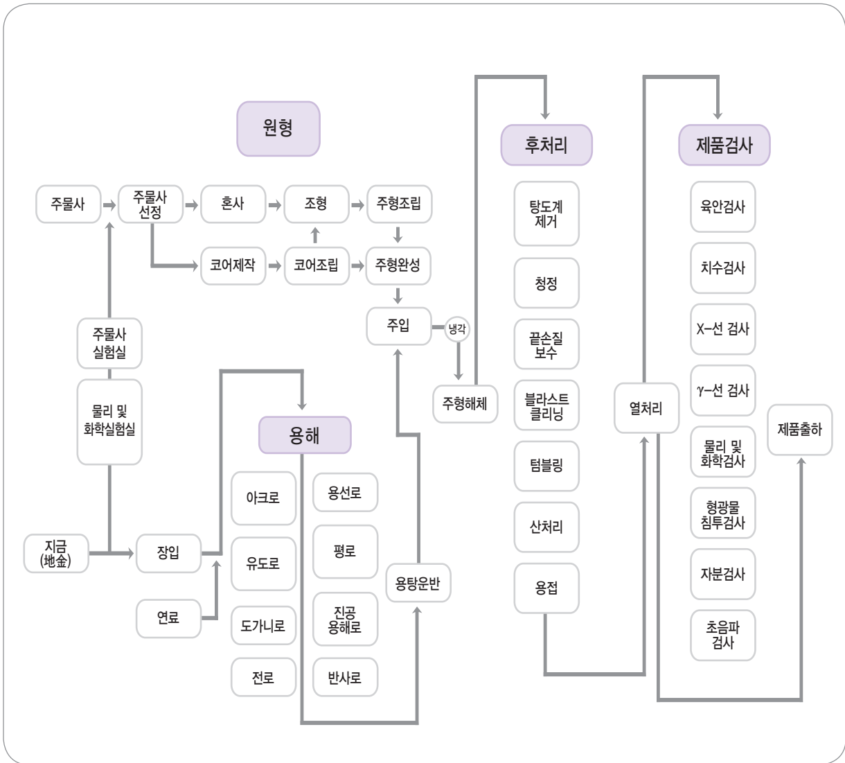
〈 주물의 제작 공정도 〉
