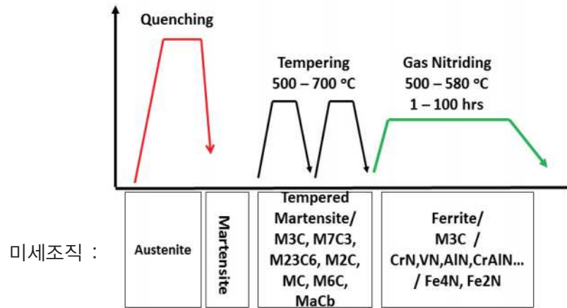
〈 Q/T 및 질화 열처리 전체 사이클 〉
