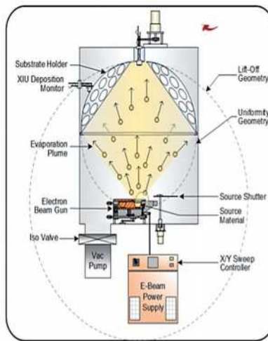
〈 E-beam 증발증착 장치 〉
