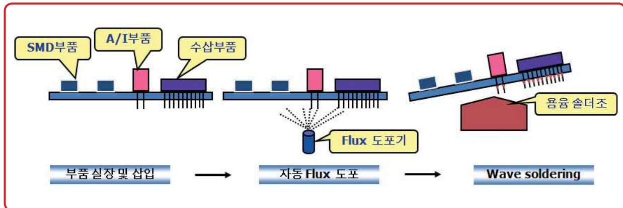
〈 웨이브솔더링 공정 모식도 〉
