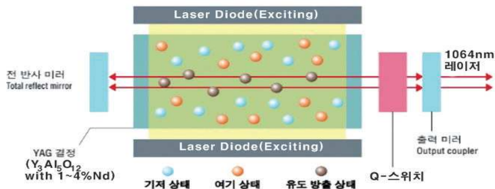
〈 Nd:YAG 레이저 작동 원리 〉
