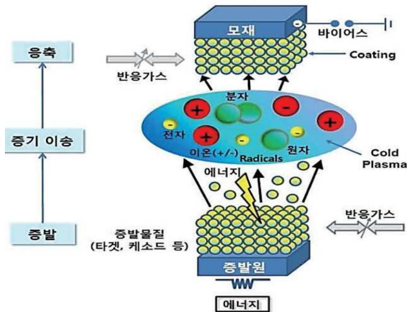
〈 건식코팅에 의한 박막 제조의 원리 〉
