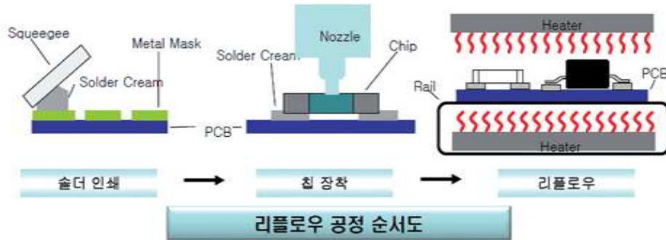
〈 표면실장 기술 주요공정 모식도 〉
