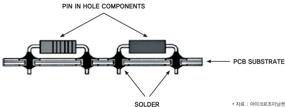
〈 PCB 단면 모식도 〉
