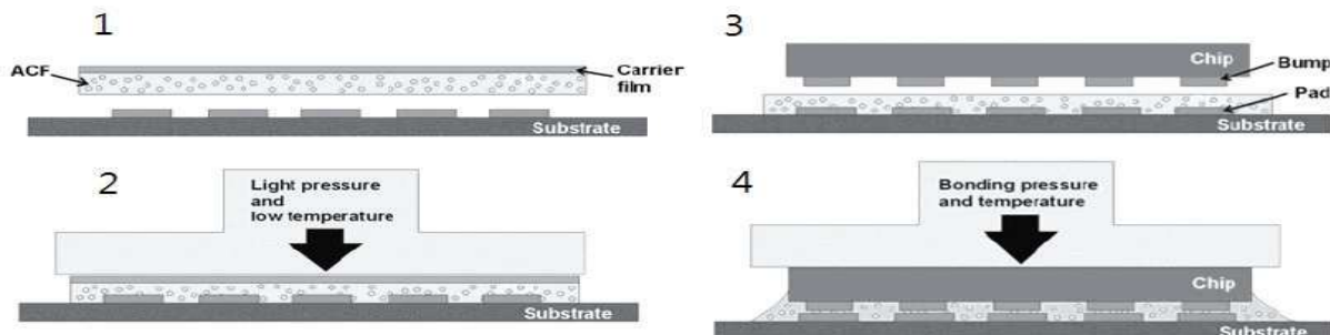
〈 일반적인 ACF 접합 공정 모식도 〉
