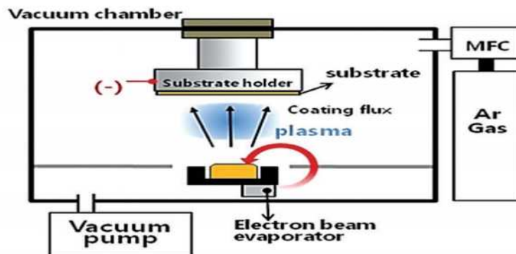
〈 이온플레이팅 증착 장치 〉
