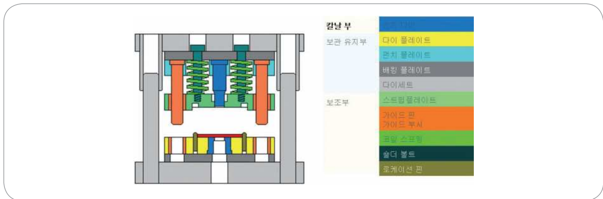
〈 프레스금형 구조 〉
