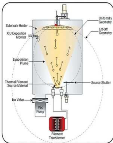
〈 열 증발증착 장치 〉
