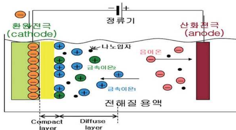
〈 전해도금 시스템의 구조 및 작동원리 〉
