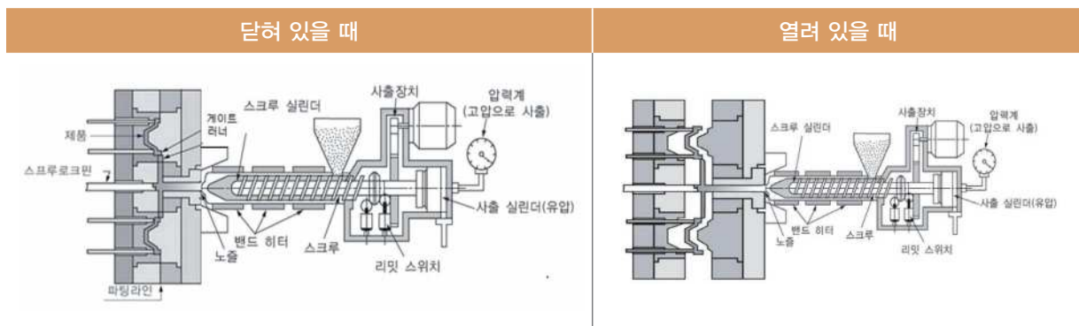
〈 사출성형 원리 〉
