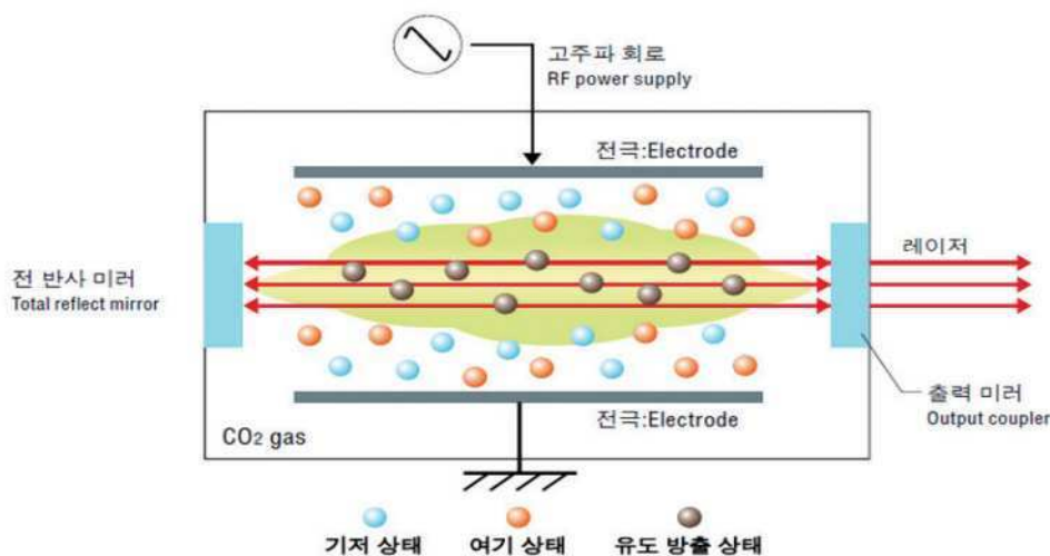
〈 CO 2 레이저 작동 원리 〉
