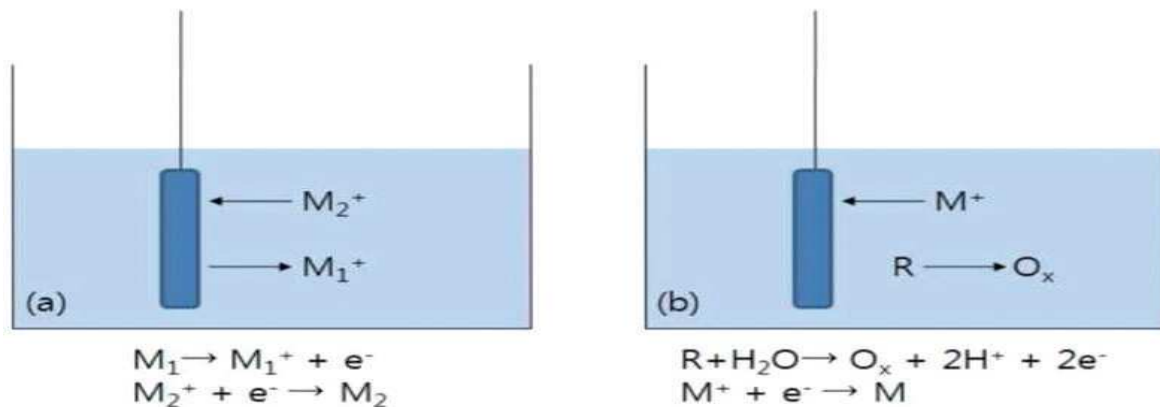
〈 치환도금(a)과 화학환원도금(b)의 작동원리 〉
