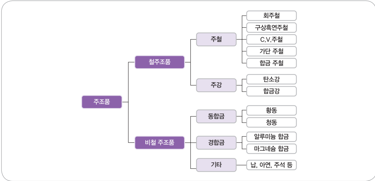
〈 사형 주조용 금속 소재(또는 합금 소재) 〉
