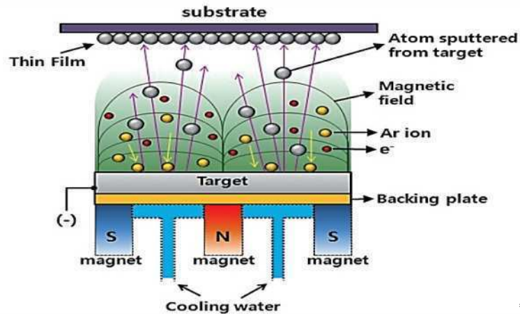
〈 스퍼터링 증착 공정 기본 단계 〉
