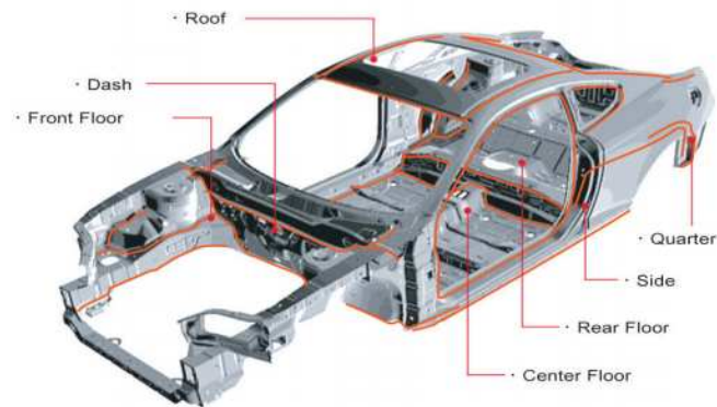
〈 구조용 접착제 차체 적용 예 〉
