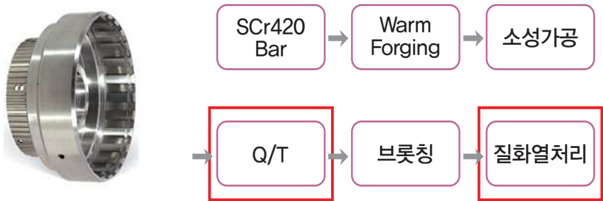
〈 애플러스 기어의 제작과정 〉
