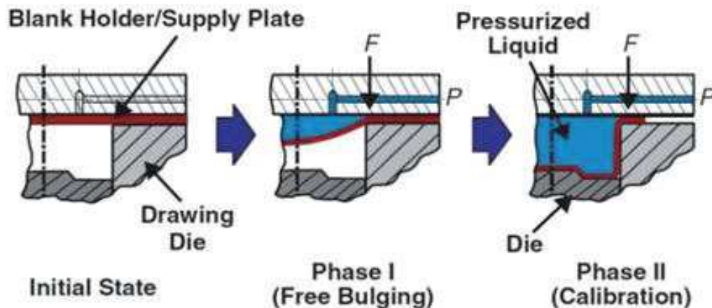
〈 시트하이드로포밍(Sheet hydroforming) 〉
