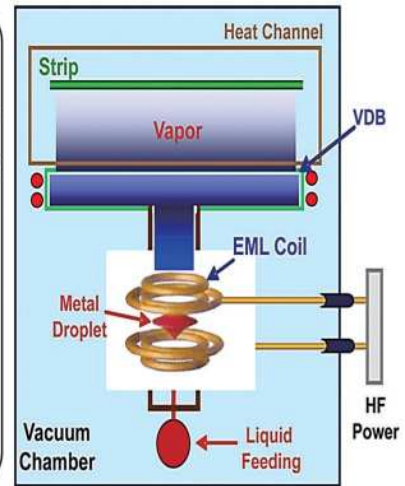
〈 도가열 증발증착 장치 〉
