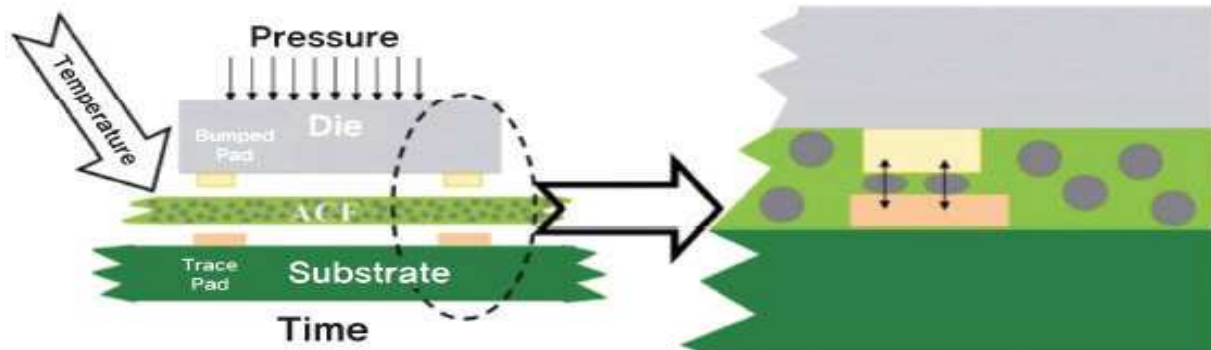
〈 ACF 접합부 모식도 〉
