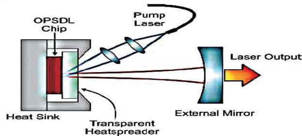
〈 Disk 레이저 작동 원리 〉
