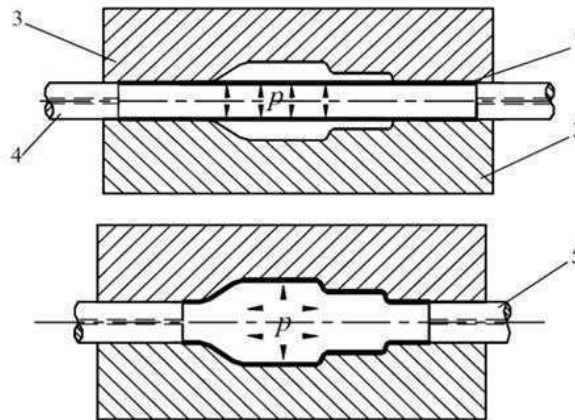
〈 튜브하이드로포밍(Tube hydroforming) 〉
